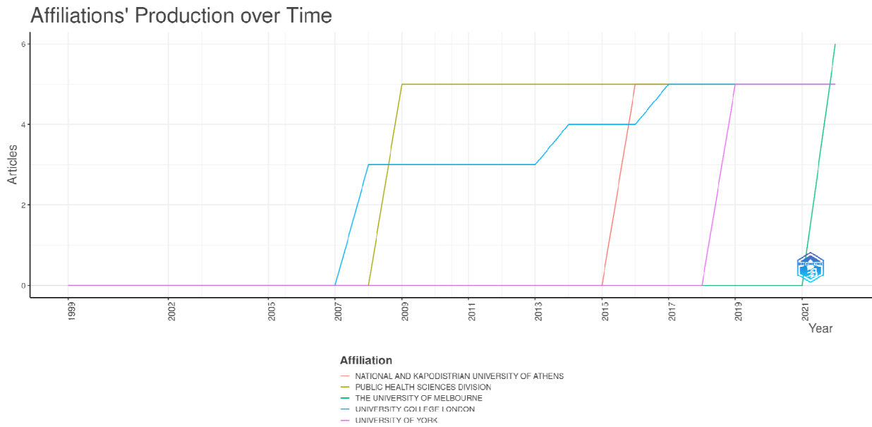
Gambar 4. Produksi Universitas waktu ke waktu.
