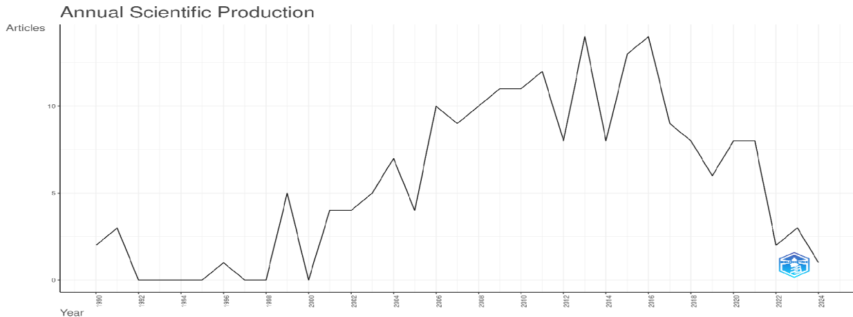
Gambar 1. Produksi Artikel Ilmiah Tahunan
